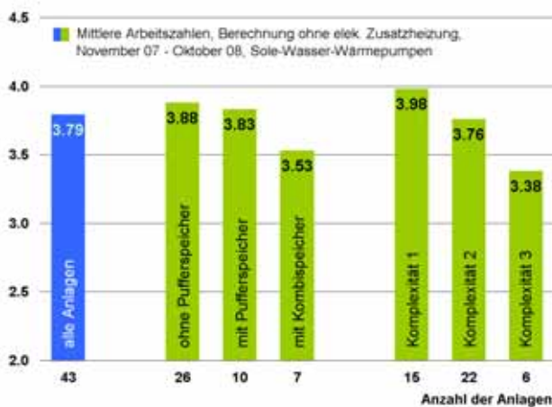
Bild 5: Abhängigkeit der Arbeitszahlen der Sole/Wasser-Wärmepumpen von der eingesetzten Speichermodelle und Komplexität der Gesamtanlage
