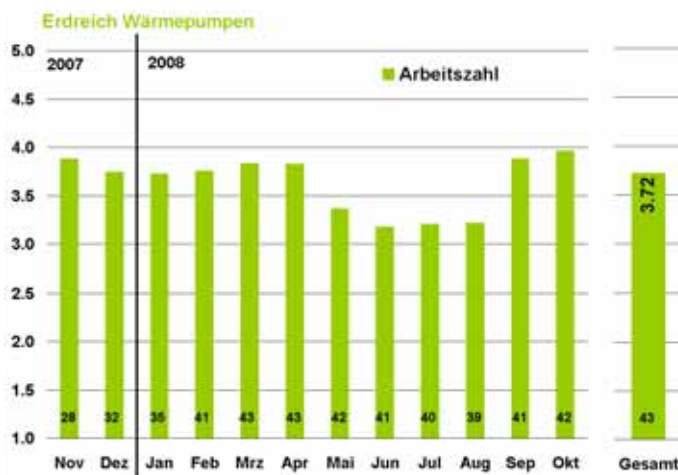
Bild 4: Mittlere Arbeitszahlen der Sole/Wasser-Wärmepumpenanlagen in dem Zeitraum vom November 2007 bis Oktober 2008 (inkl. Elektrozusatzheizung)
